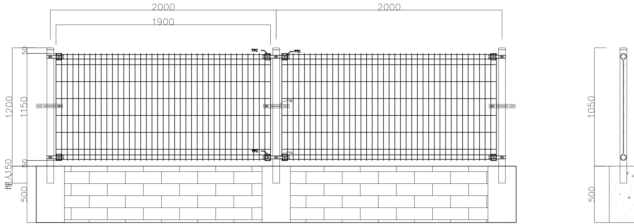
鍍鋅鋼網圍籬立面圖
