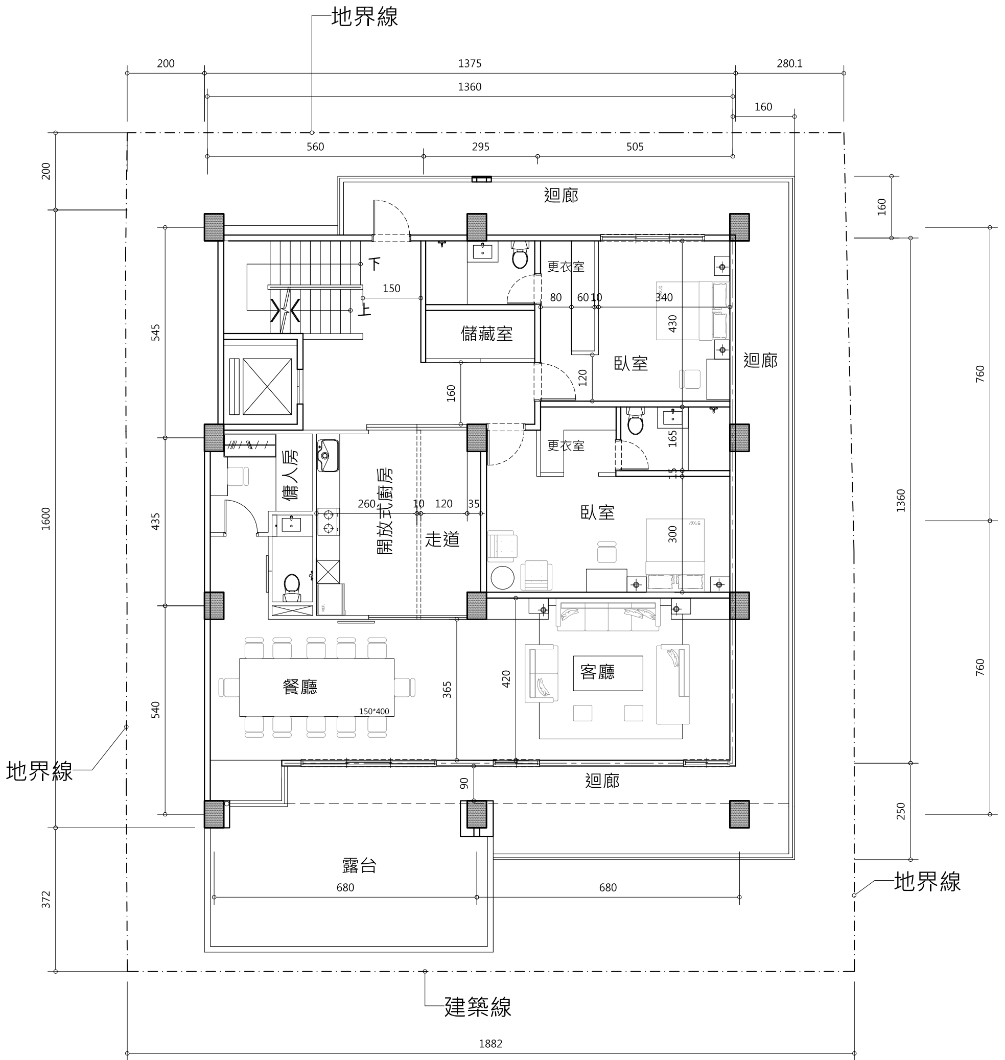
2 二樓平面圖 Scale=1/100
