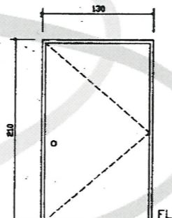
⑩ 烤漆鐵板門 SCALE 1/30
