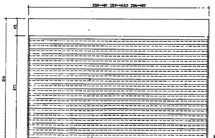
⑭ 電動不銹鋼捲門 SCALE 1/30
