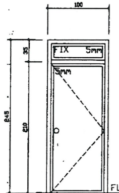
⑦ 鋁門 SCALE 1/30
