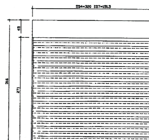
⑮ 電動不銹鋼捲門 SCALE 1/30
