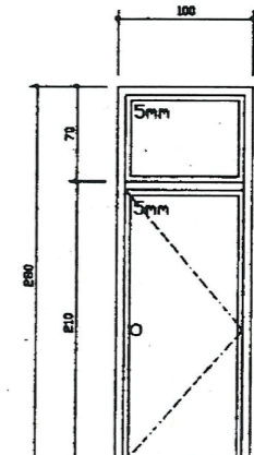
⑫ 鋁門 SCALE 1/30
