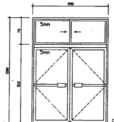
⑪ 鋁門 SCALE 1/30
