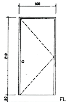
⑧ 烤漆鐵板門 SCALE 1/30
