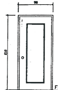
⑤ 玻化銅門 SCALE 1/30 (圖式另定)
