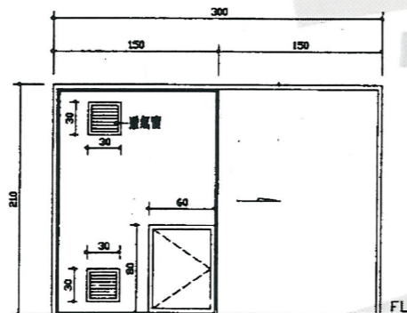
⑨ 烤漆鐵板門 SCALE 1/30
