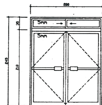
⑥ 鋁門 SCALE 1/30
