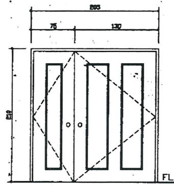
① 玻化銅門 SCALE 1/30 (乙種防火門) (圖式另定)
