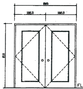
② 玻化銅門 SCALE 1/30 (乙種防火門) (圖式另定)
