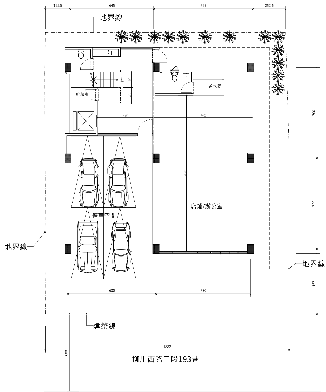
1 一樓平面圖 Scale=1/100
