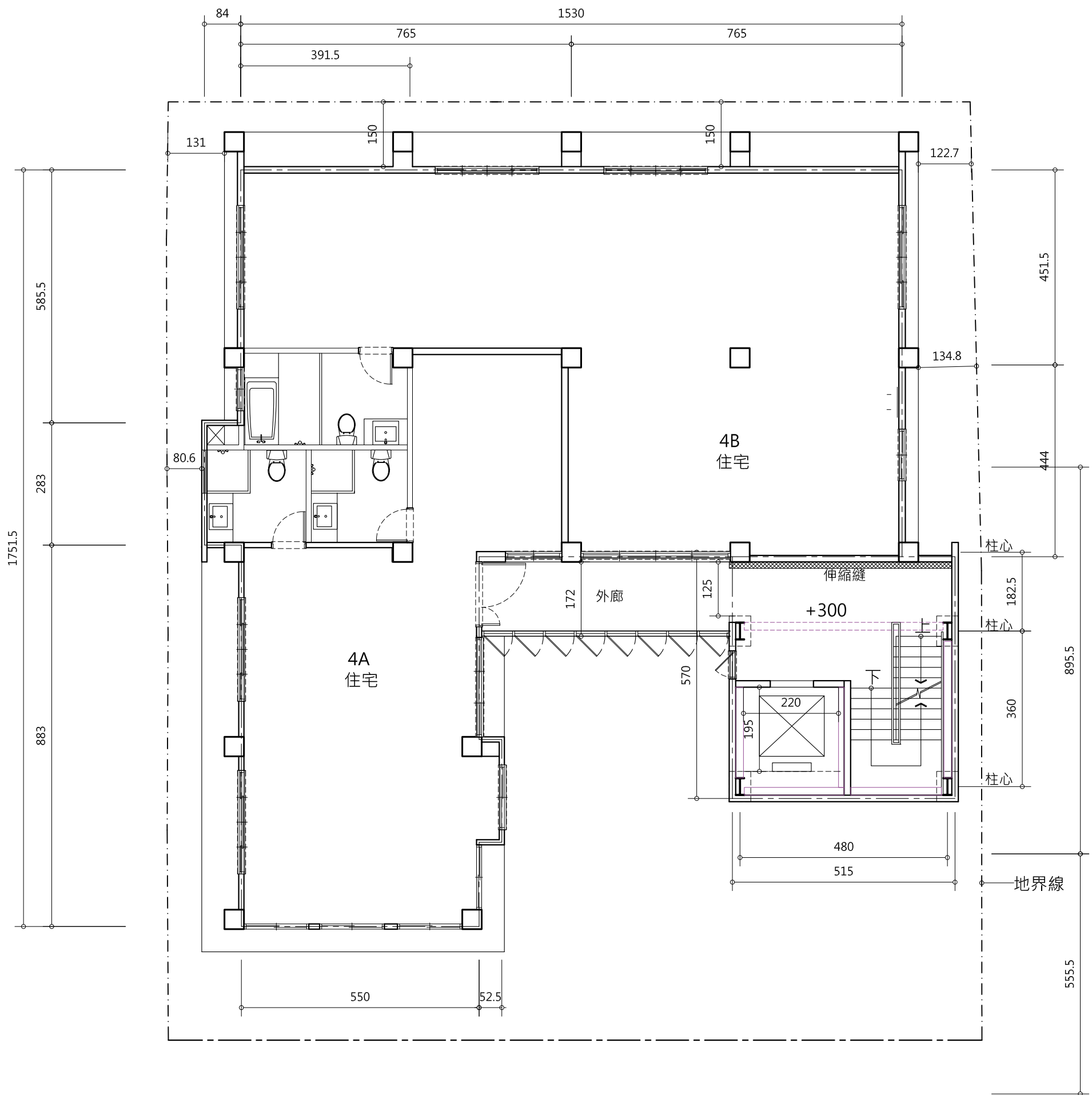
四層平面圖 scale=1/100
