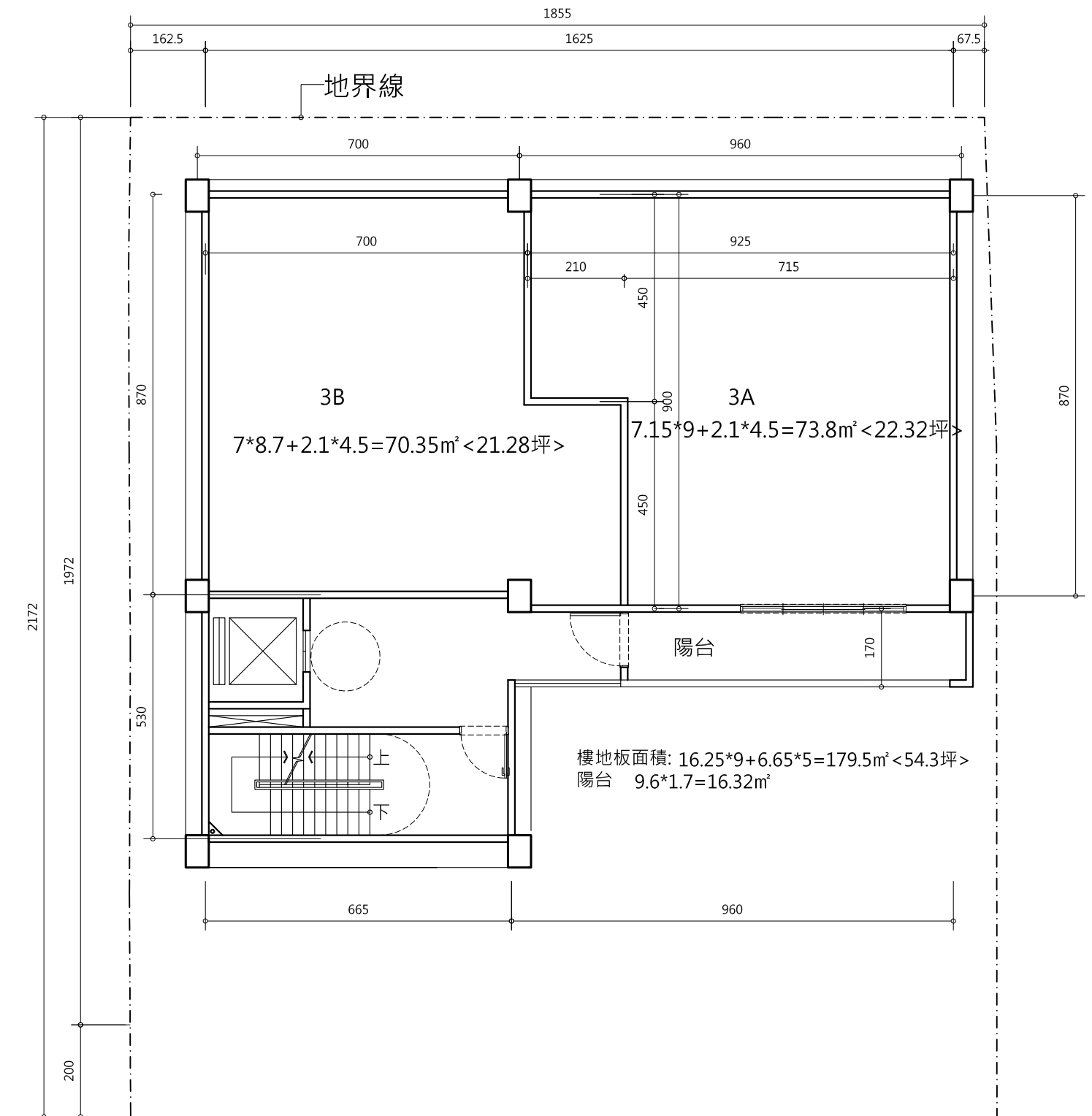
4 三樓平面圖 Scale=1/150
