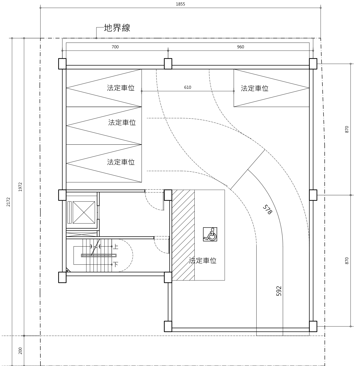
1 地下一層平面圖 Scale=1/150
